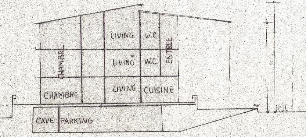
COUPE MAISON MULTIFAMILIALE ech. 1.250
